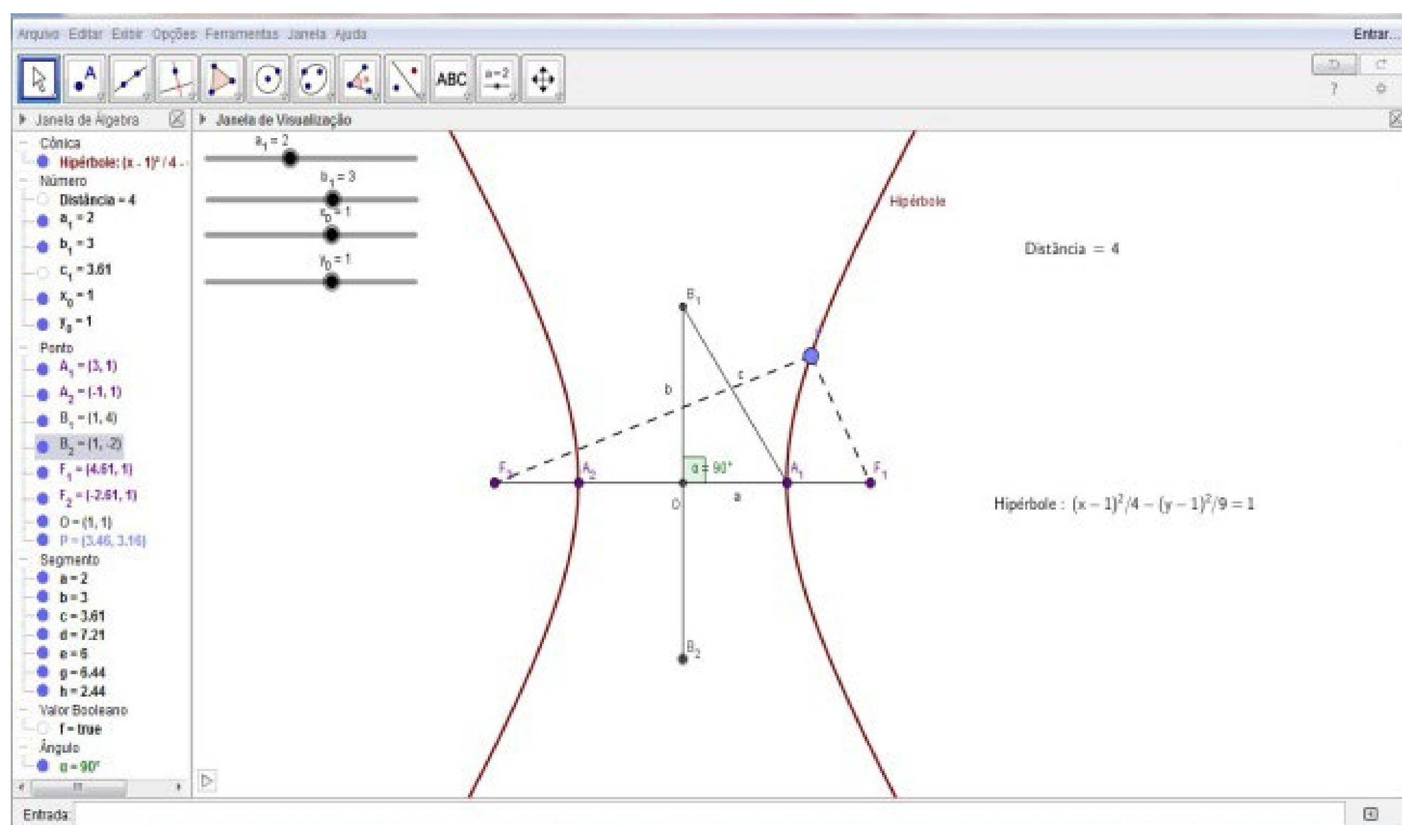
Figura 2 - Gráfico da Hipérbole no software Geogebra Fonte: Santos (2016)
